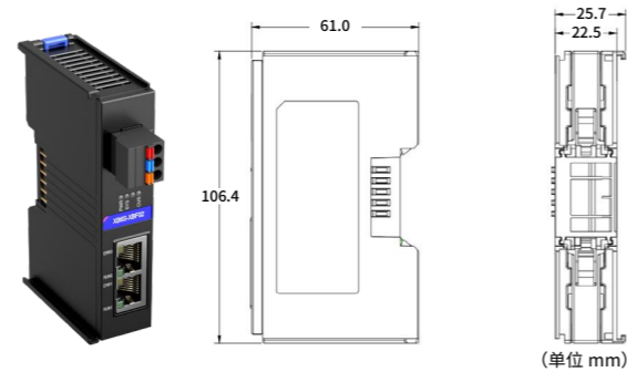
XB6S-XBF02 尺寸图
