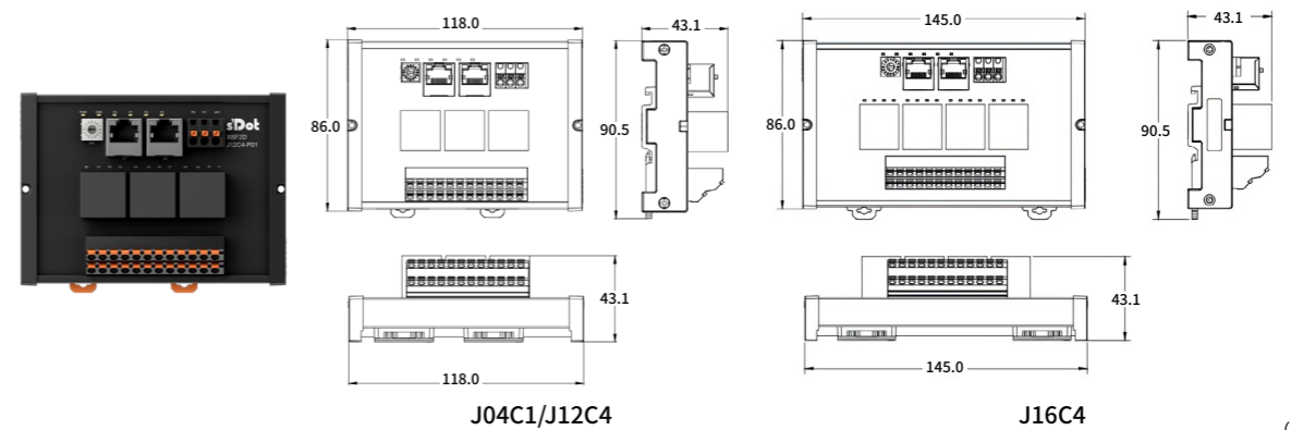
XBF2D 系列尺寸图
