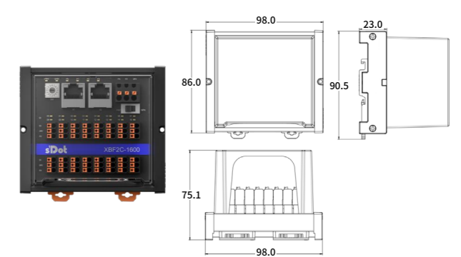
尺寸图 (含防尘罩)
