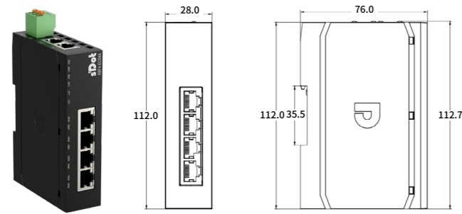
XBF4 系列耦合器尺寸图
