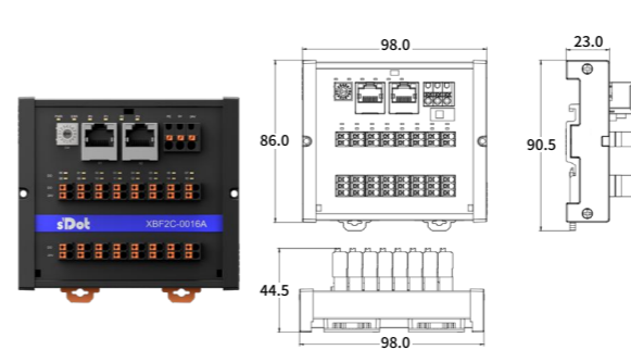
XBF2C 系列尺寸图 (不含防尘罩)
