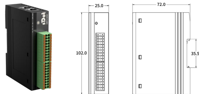
XBF4 系列尺寸图
