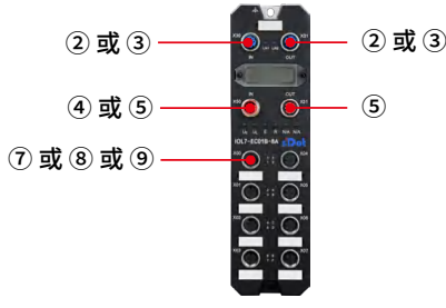
IO-Link 主站
