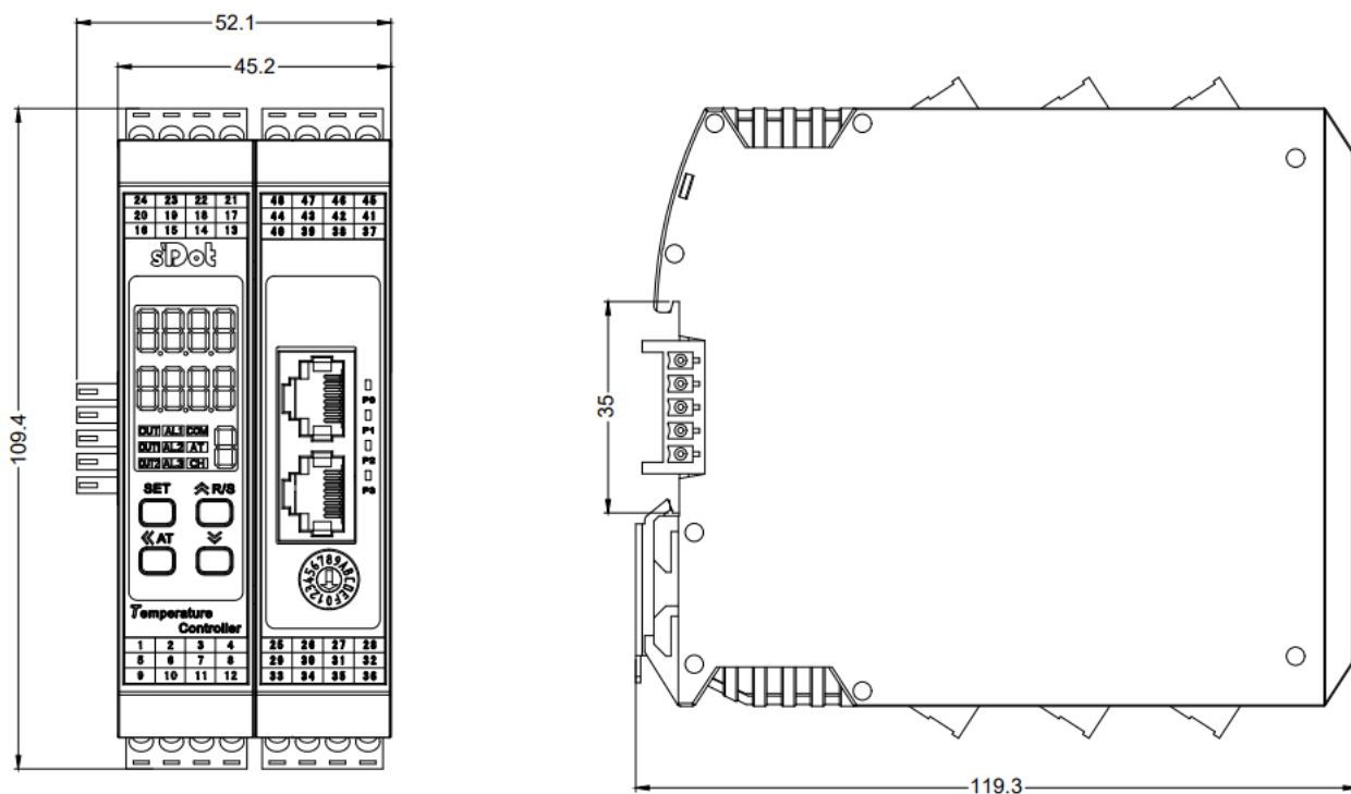
外形规格 (单位 mm)
