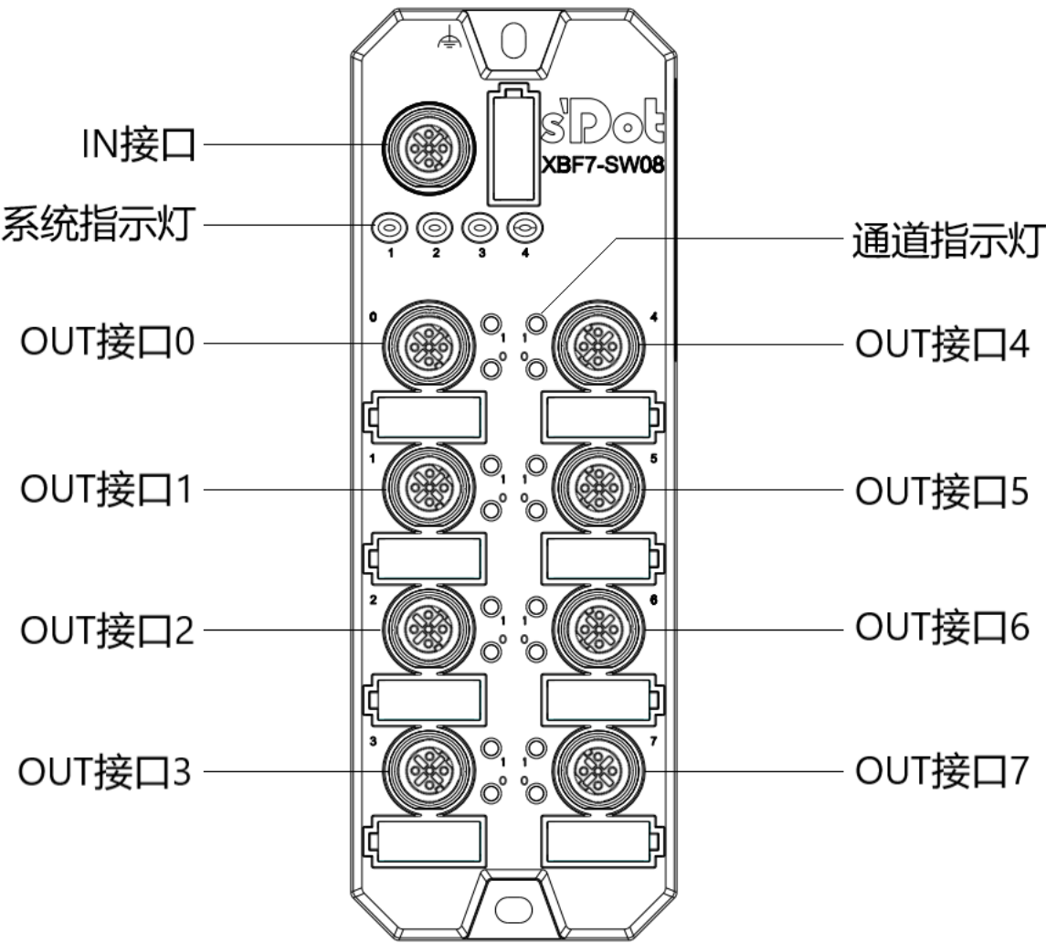
产品各部位名称
