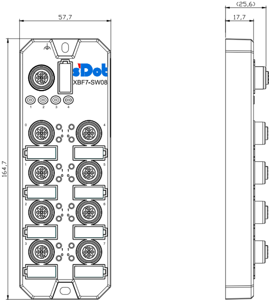
外形规格 (单位 mm)
