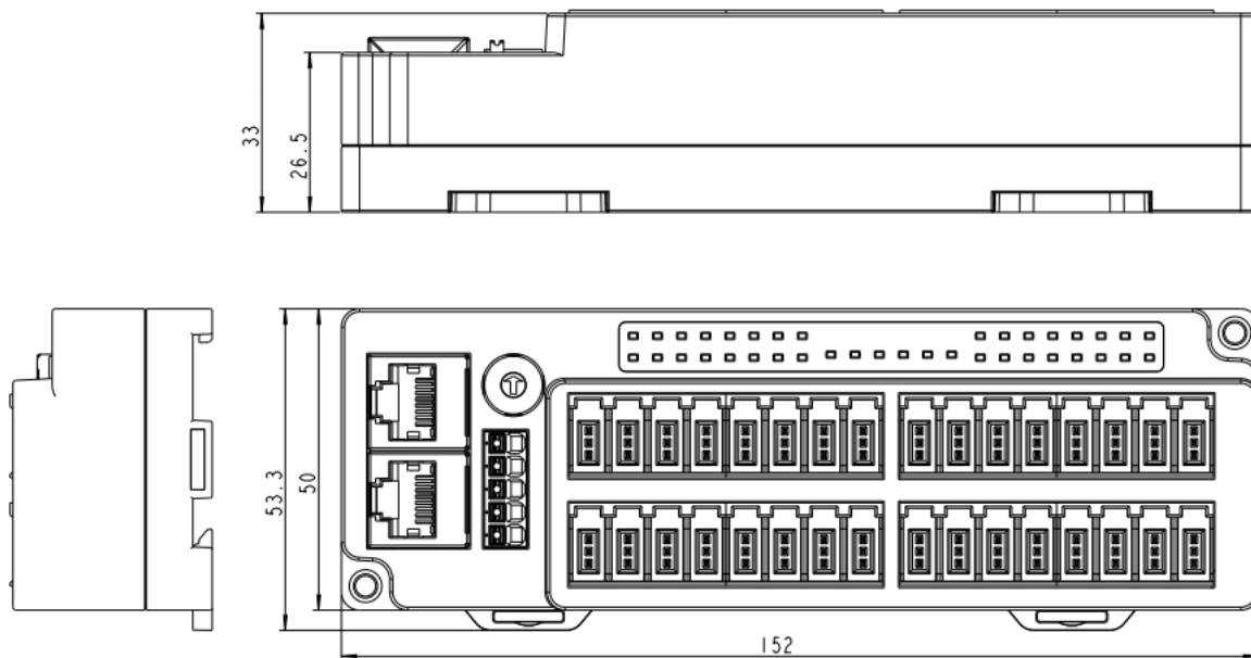
32 通道 I/O 模块外形规格 (单位 mm)
