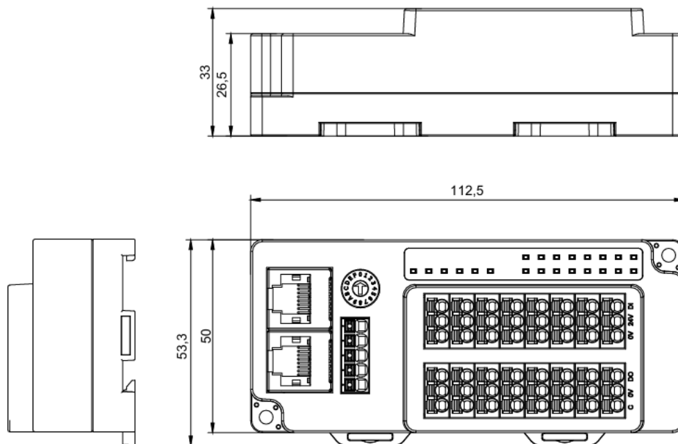
16 通道 I/O 模块外形规格 (单位 mm)
