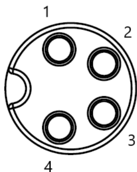
I/O 扩展接口连接视图 (A-code, 4Pin, 孔端)
