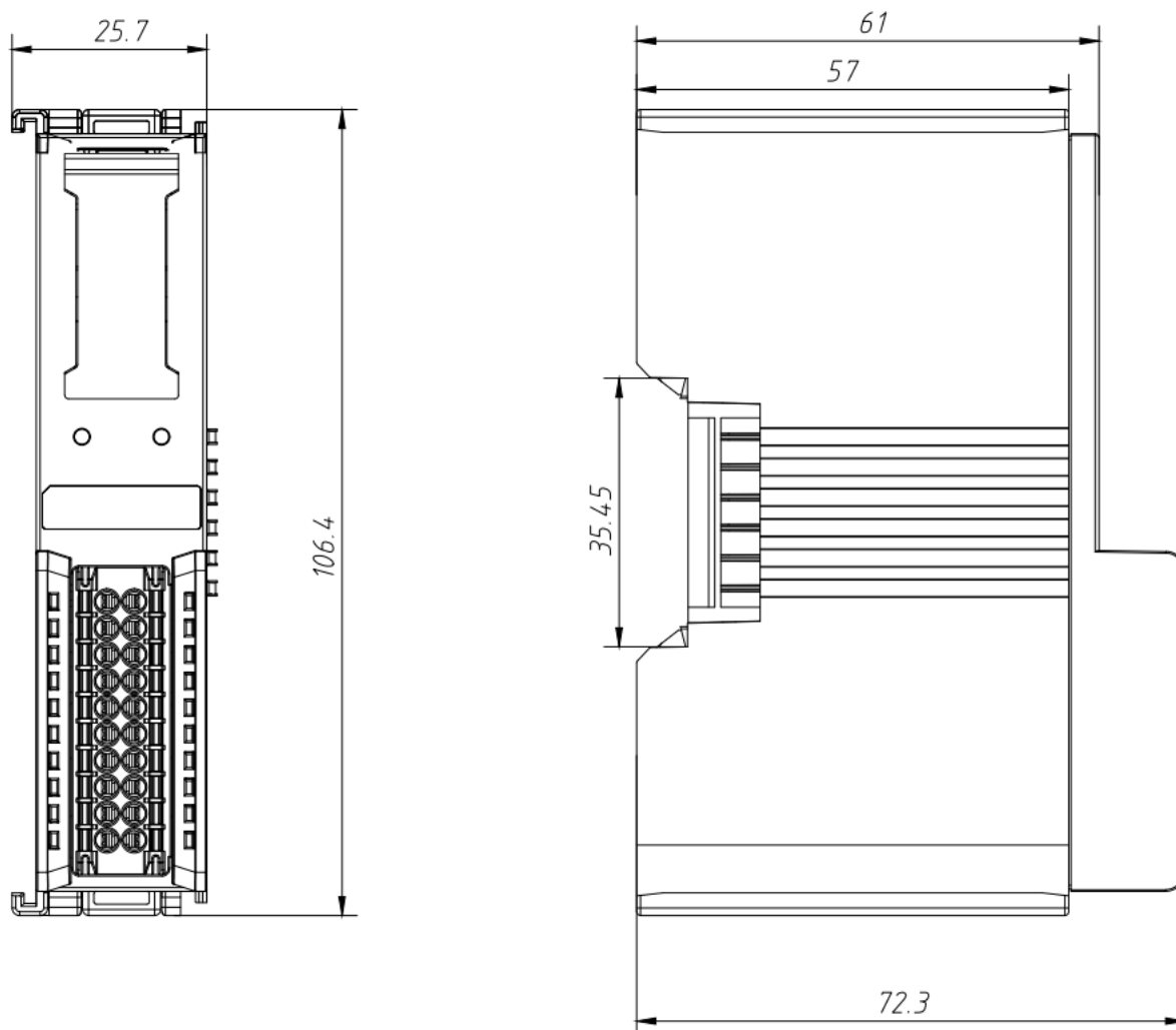
16 通道数字量 I/O 模块外形规格 (单位 mm)
