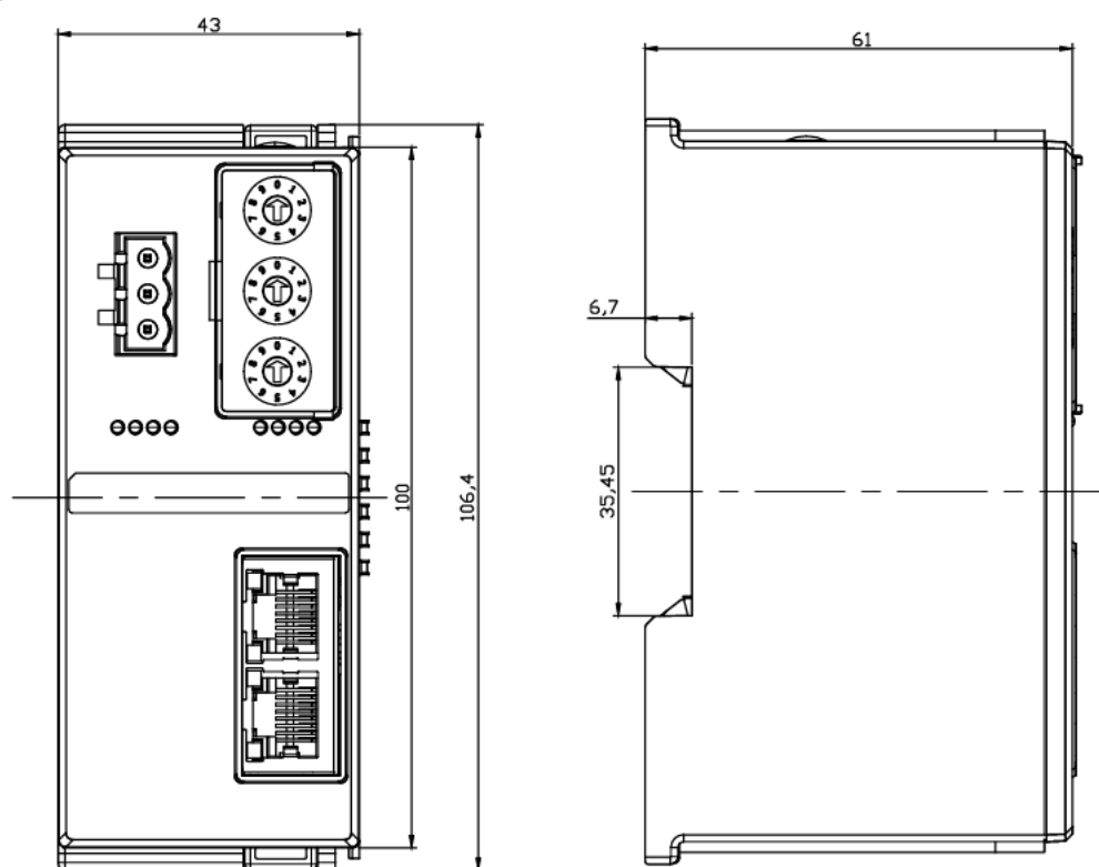
耦合器外形规格 (单位 mm)
