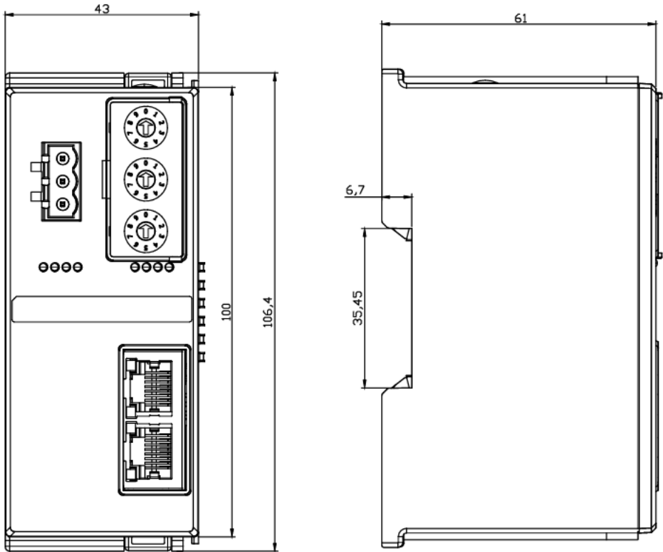
耦合器外形规格（单位 mm）
