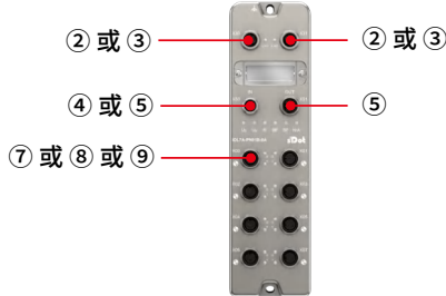
IO-Link 主站
