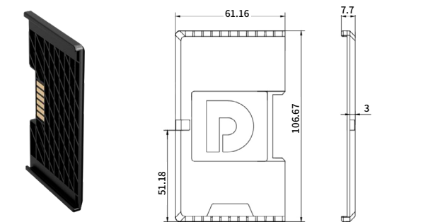
XB6S 终端盖板尺寸图
