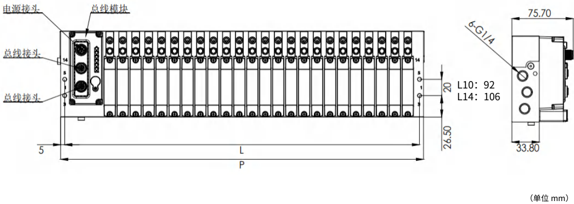
C3 系列阀岛尺寸图
