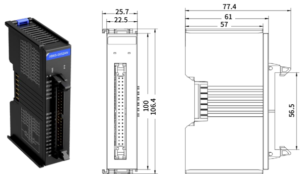
XB6S MIL 连接器型模块尺寸图
