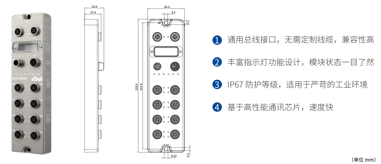
IP67 总线 I/O 及尺寸图
