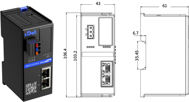
XB6S 耦合器尺寸图
