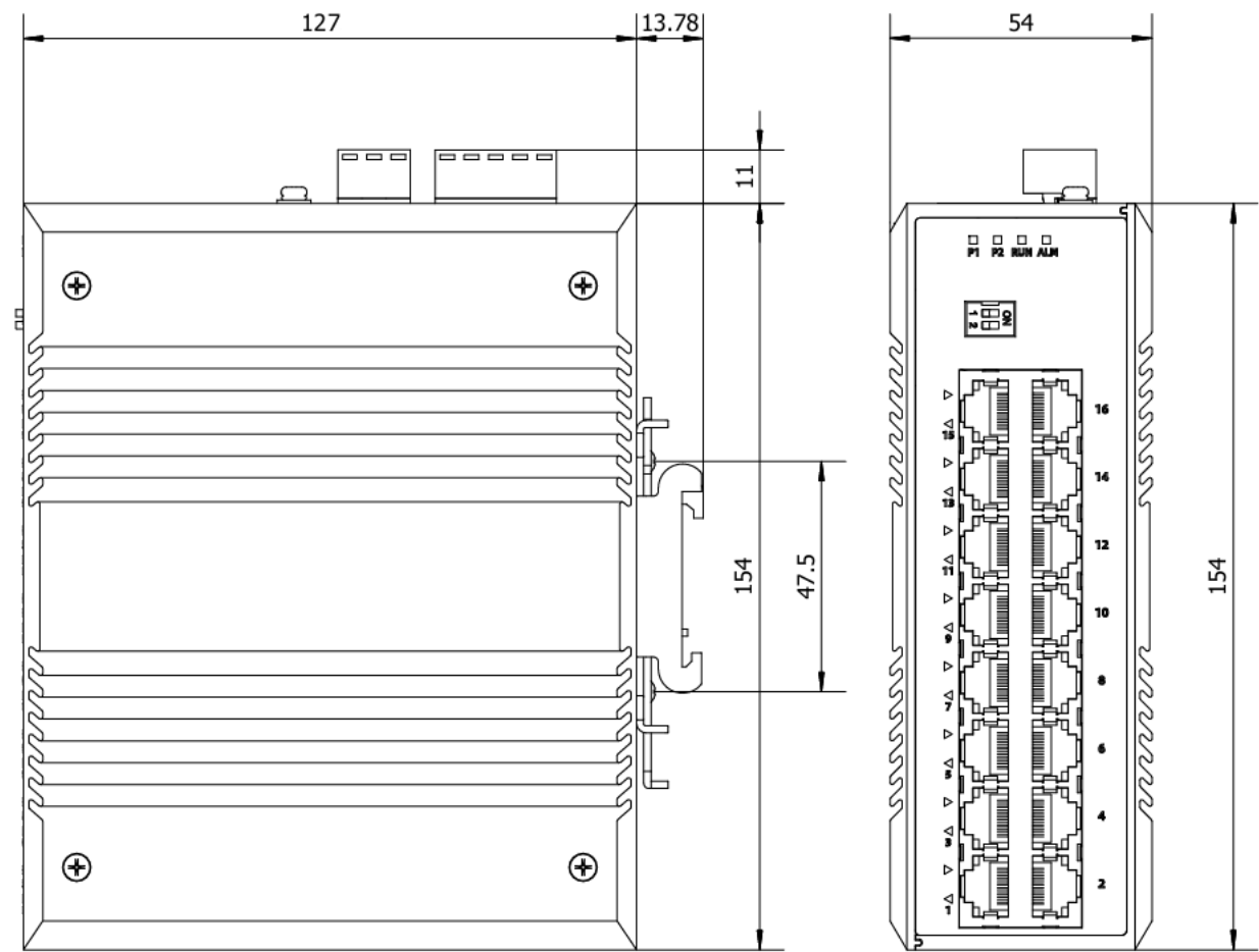
外形规格 (单位 mm)
