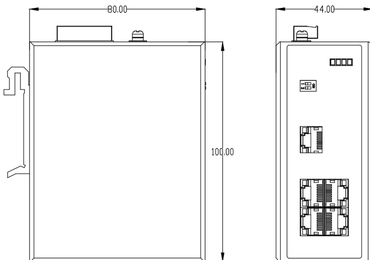
外形规格 (单位 mm)
