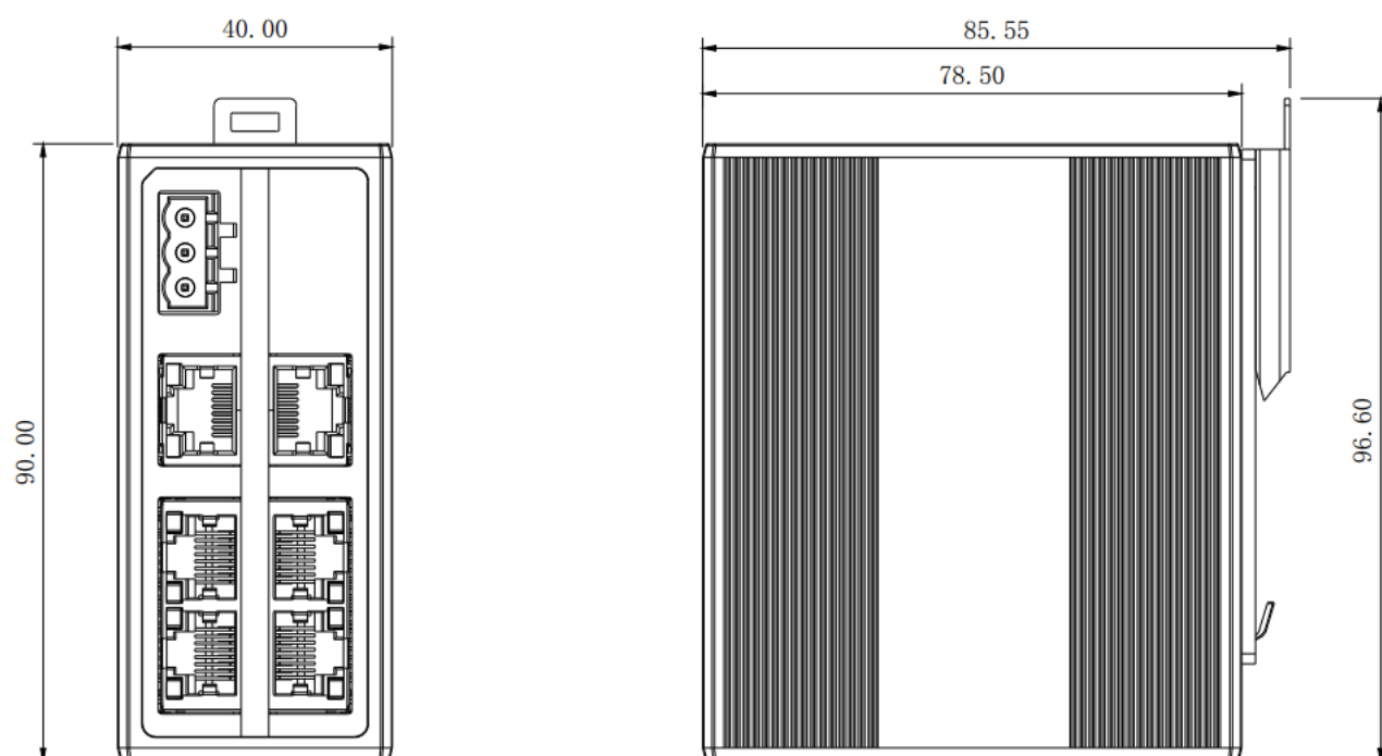
外形规格 (单位 mm)
