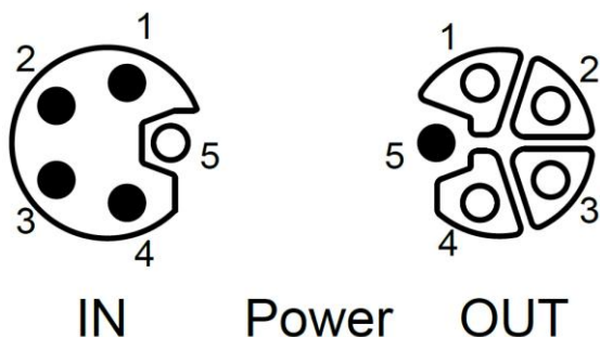
电源接口连接视图 (M12-L, 针端&amp;孔端)
