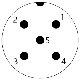
IO-Link 接口连接视图 (Class-B 端口, 针端) 定义说明
