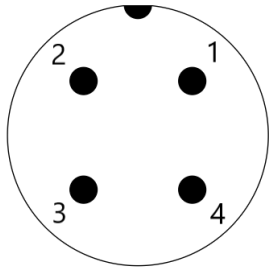
IO-Link 接口连接视图 (Class-A 端口, 针端) 定义说明
