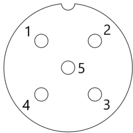
I/O 接口连接视图 (M12, 孔端) 定义说明
