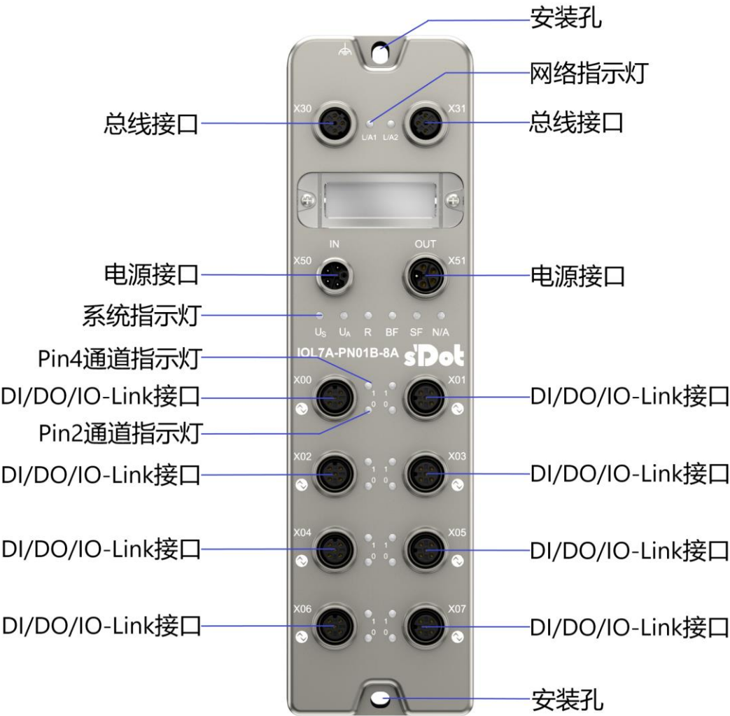
产品各部位名称
