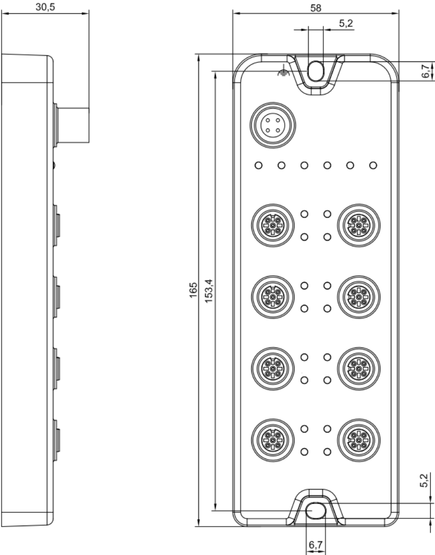
外形规格 (单位 mm)
