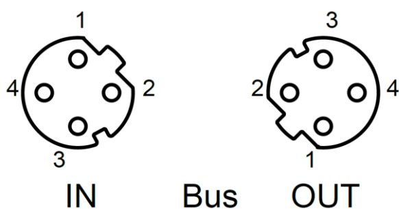
总线接口连接视图 (M12, D-code, 孔端)
