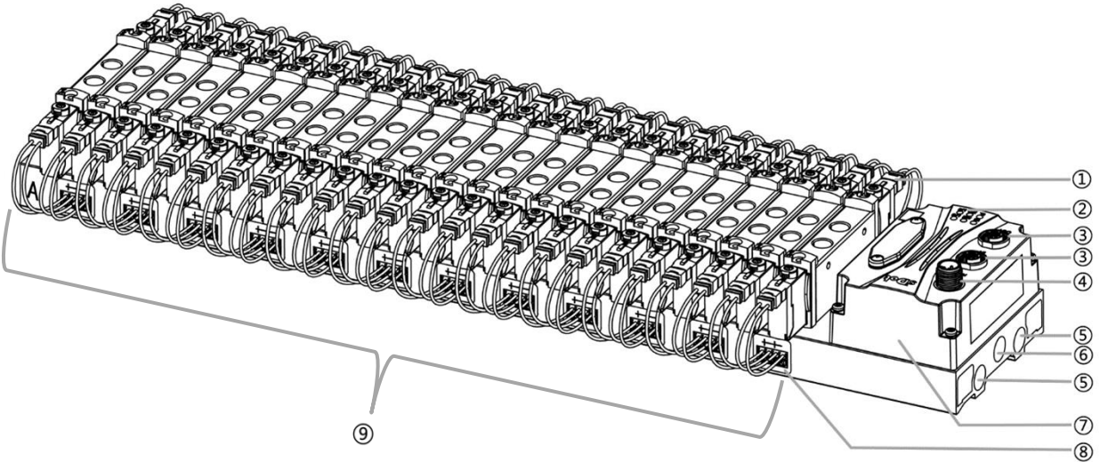
产品各部位名称和功能描述
