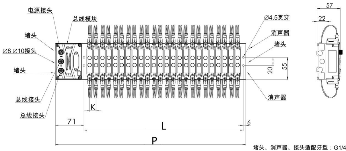
外形规格 (单位 mm)
