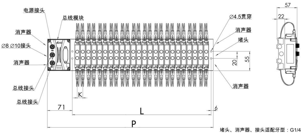
外形规格 (单位 mm)
